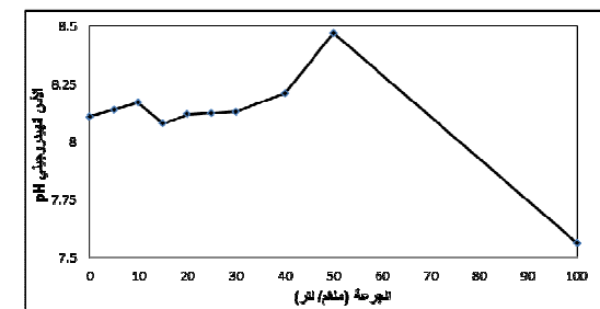
شكل (٤): العلاقة بين جرعة إضافة البوليمر والأس الهيدروجيني للراشح عند نسبة ٠,٠% EMI
