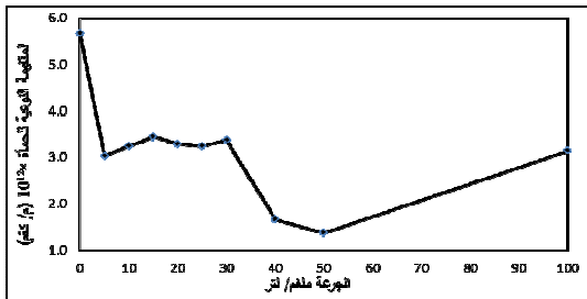
شكل (٢): العلاقة بين جرعة إضافة البوليمر ومقاومة الحمأة النوعية للترشيح عند نسبة ٠,٠٠٠ EM1
