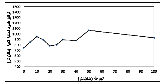
شكل (٣): العلاقة بين جرعة إضافة البوليمر والمواد الصلبة الكلية للراشح عند نسبة ٠,٠% EMI
